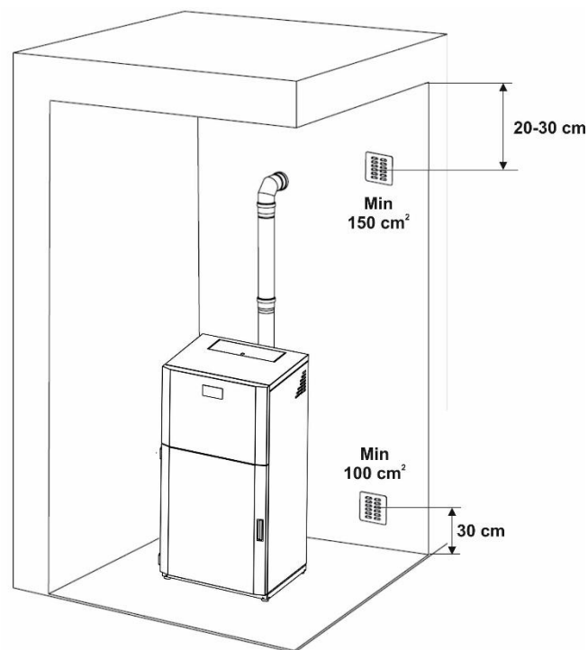
Fig. 2 Deschideri admisie aer
